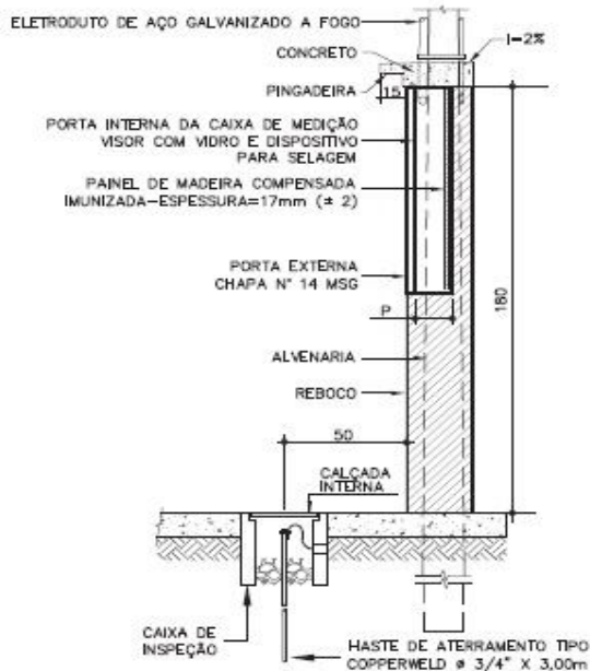
CORTE A-A SEM ESC.
